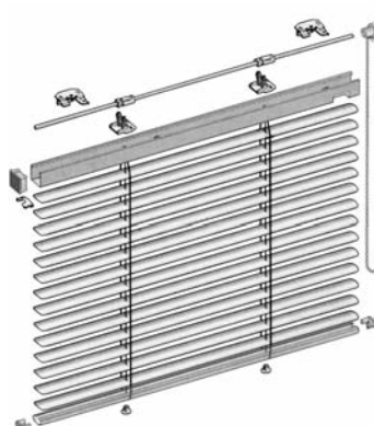
Monocomando " Soline " (sistema a catenella)
