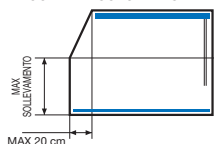
H - ORIENTAMENTO + SOLLEVAMENTO COMANDI SOLO A DESTRA
