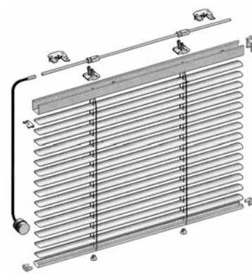
Monocomando " Uniflex " (sistema infravetro)
